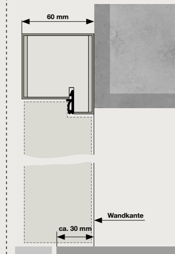
Blendrahmen 60 x 67 mm für stumpfe Türen - beidseitig flächenbündig
